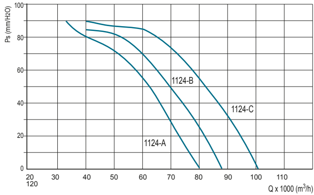
DUCT-M 1120 - 4 poles
